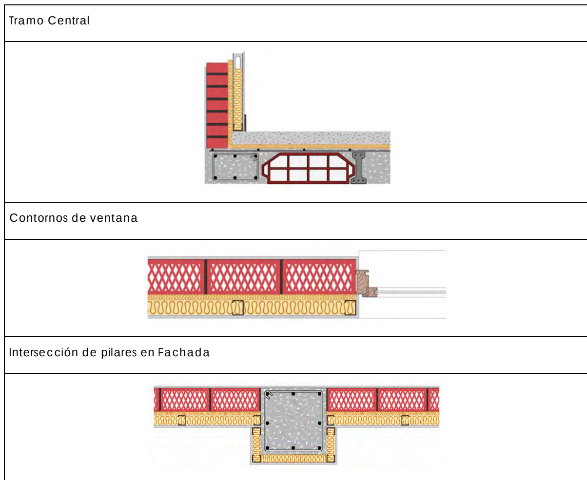
Figura 7. Detalles constructivos.
