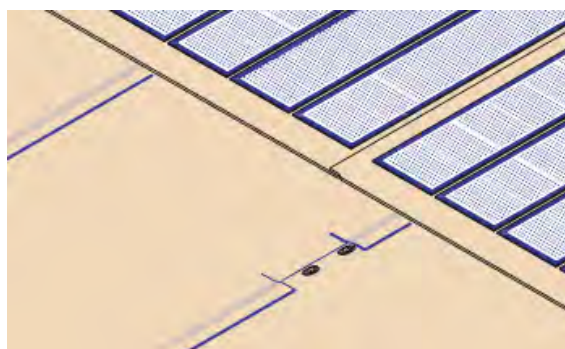
Figura 6. Sistema Sarnafast
